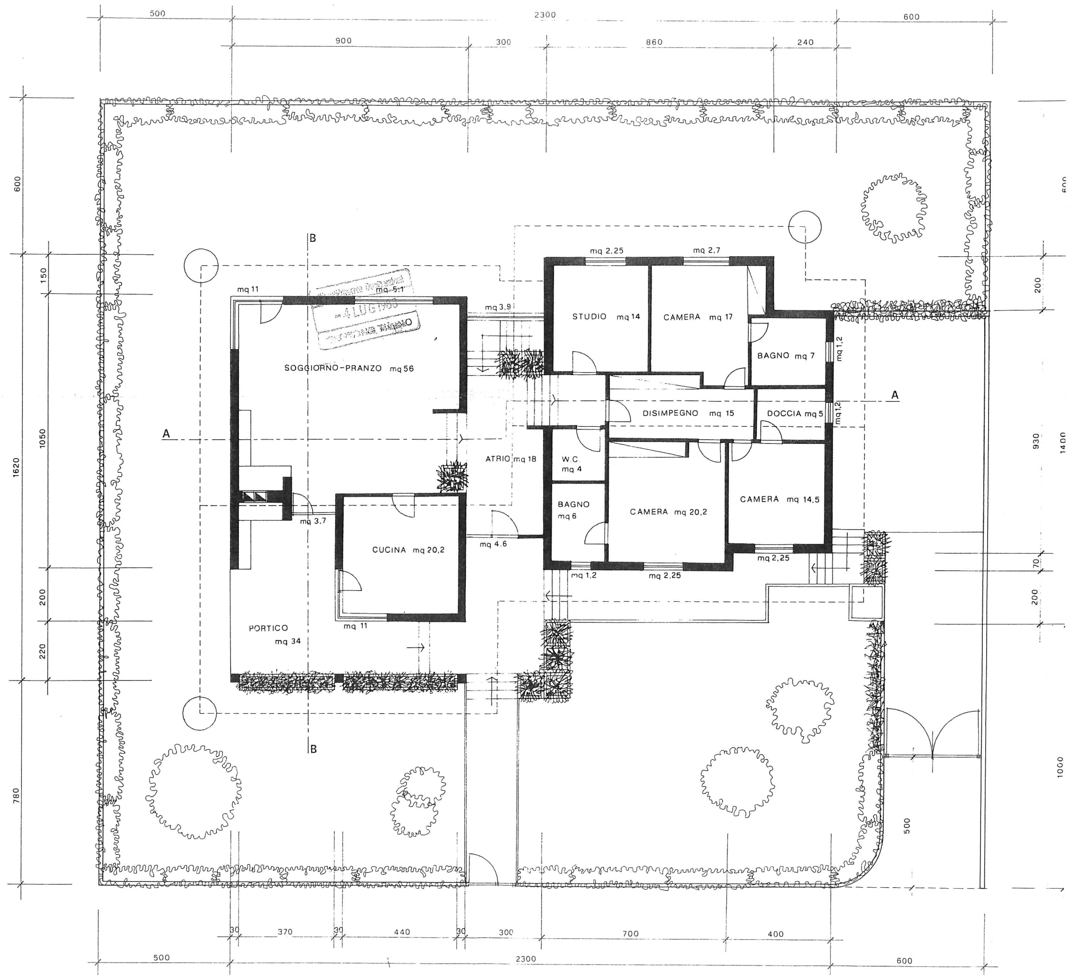
PIANTA PIANO TERRENO E RIALZATO
